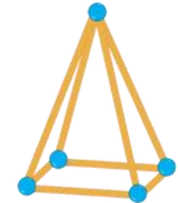
Pirámide cuadrangular
