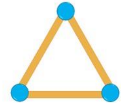
Triángulo
