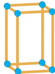
Prisma cuadrangular
